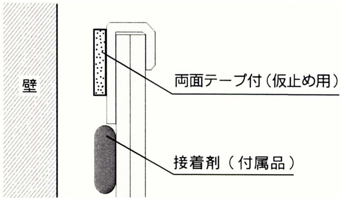
■F15、F33詳細図例
